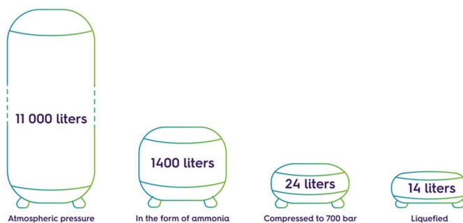
Obrázek 1: Přehled technologií skladování vodíku 1
